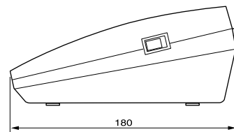
(側面)
