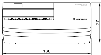
(正面)
