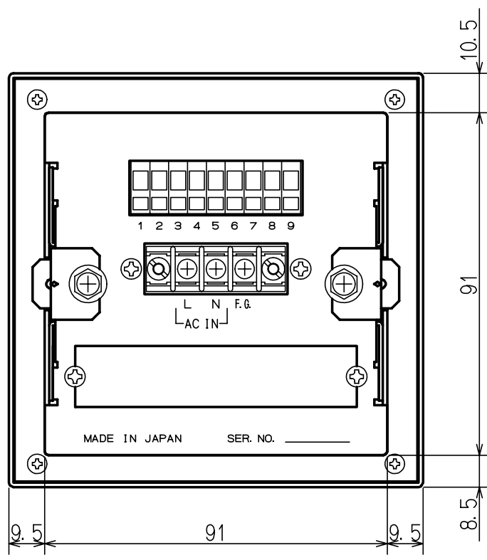
【背面】
