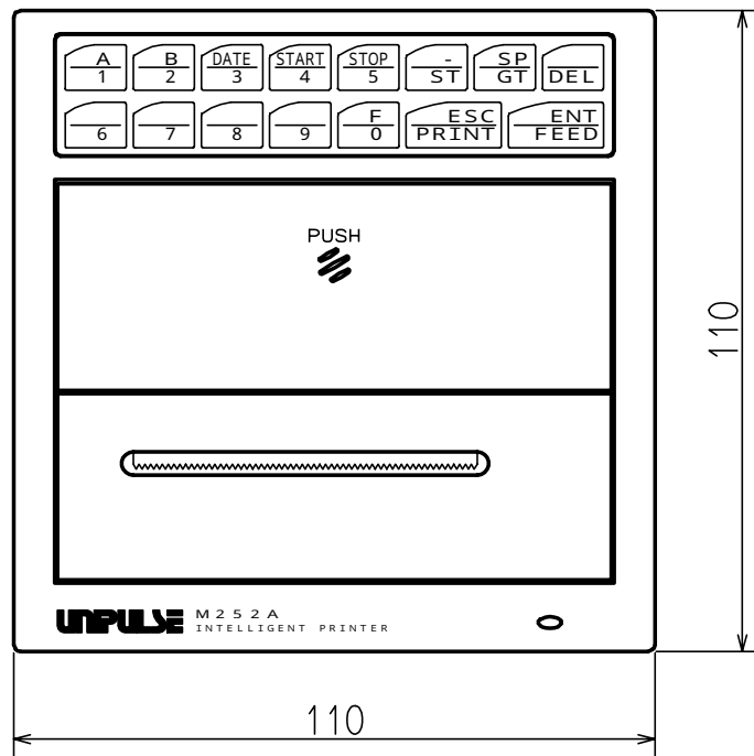
【正面】
