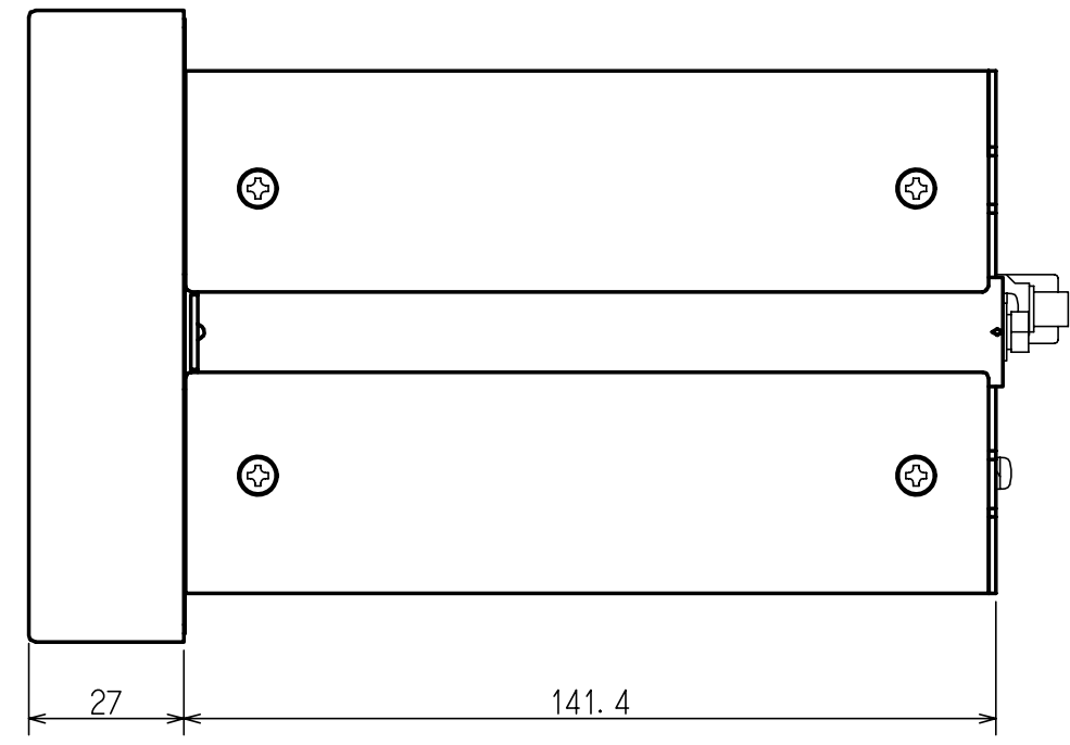
【側面】
